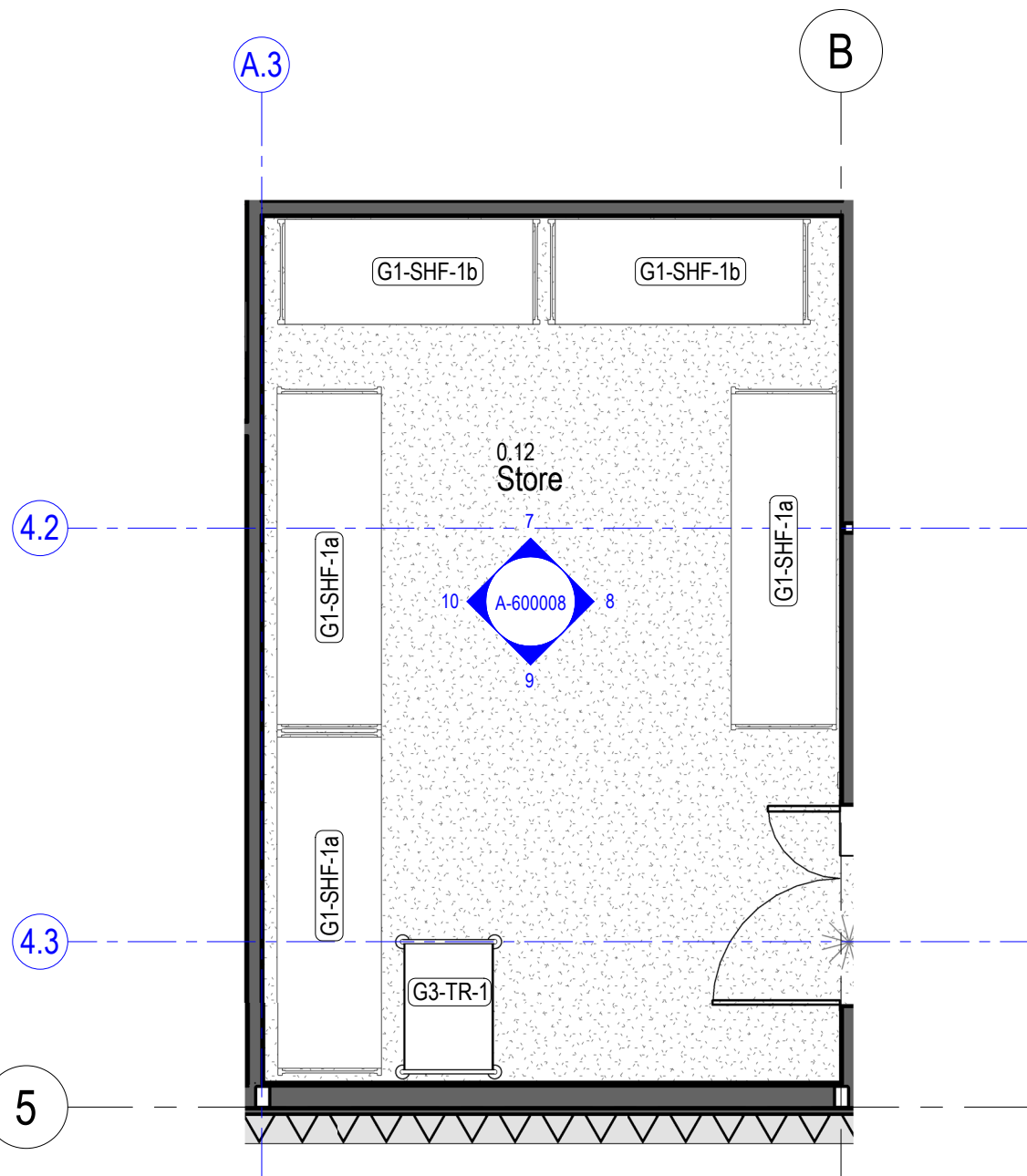
6 0.12 - Store - Plan 1 : 50
