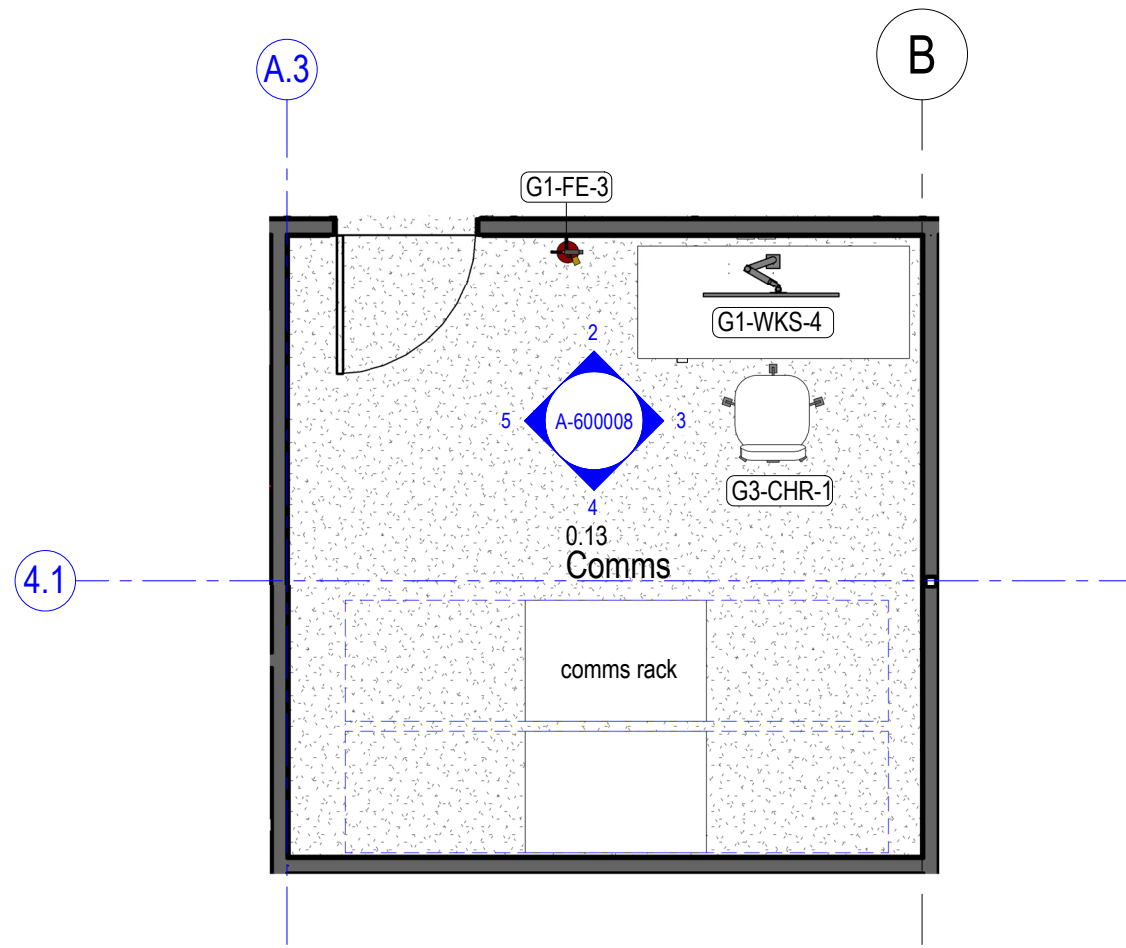
1 0.13 - Comms - Plan 1 : 50
